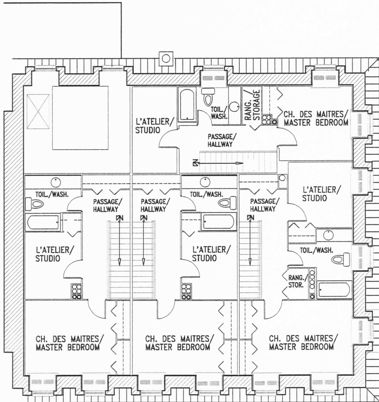
PLAN DU QUATRIÈME ÉTAGE / FOURTH FLOOR PLAN
