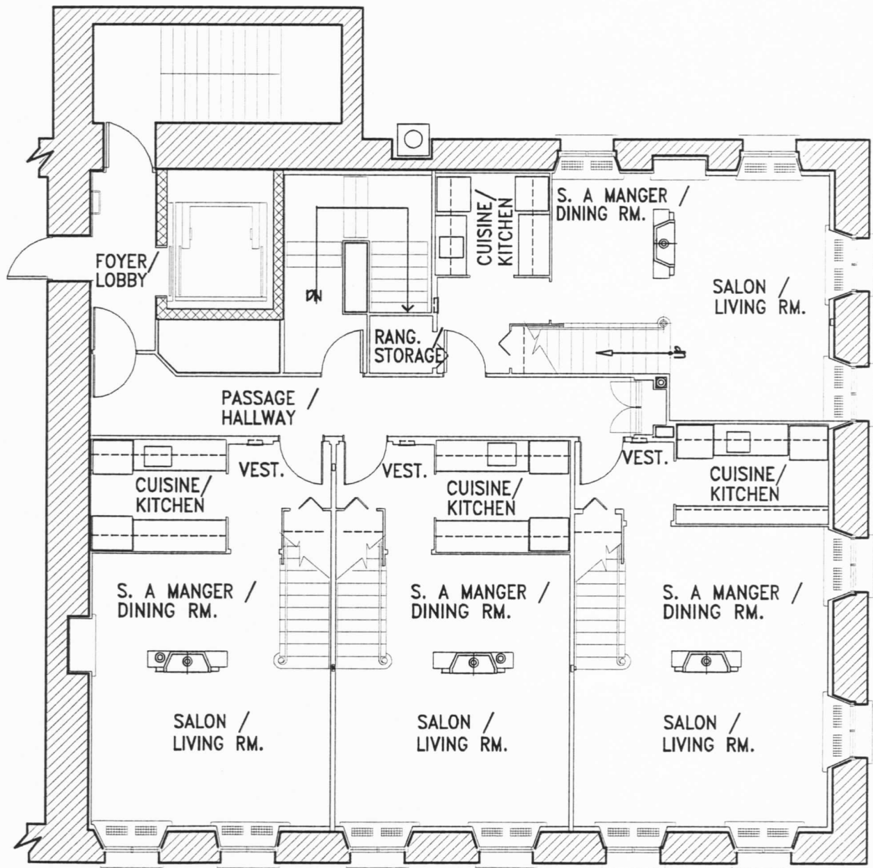
PLAN DU TROISIÈME ÉTAGE / THIRD FLOOR PLAN
