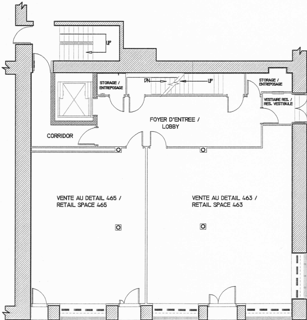
PLAN DU REZ DE CHAUSSÉE GROUND FLOOR PLAN
