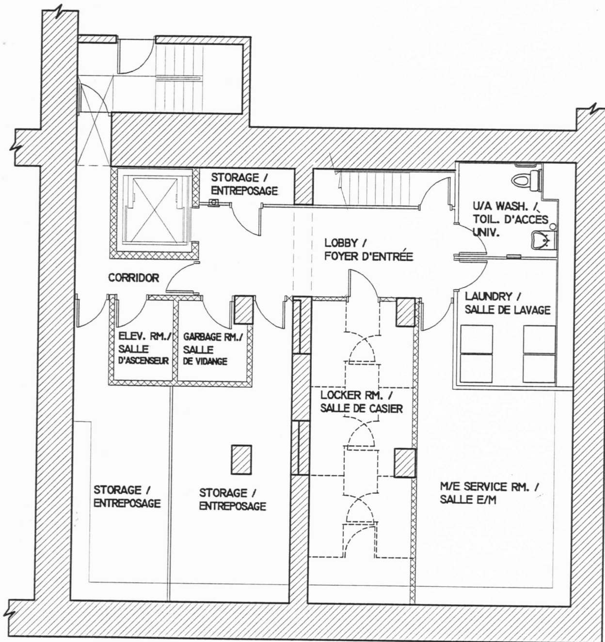
PLAN DU SOUS-SOL BASEMENT PLAN
