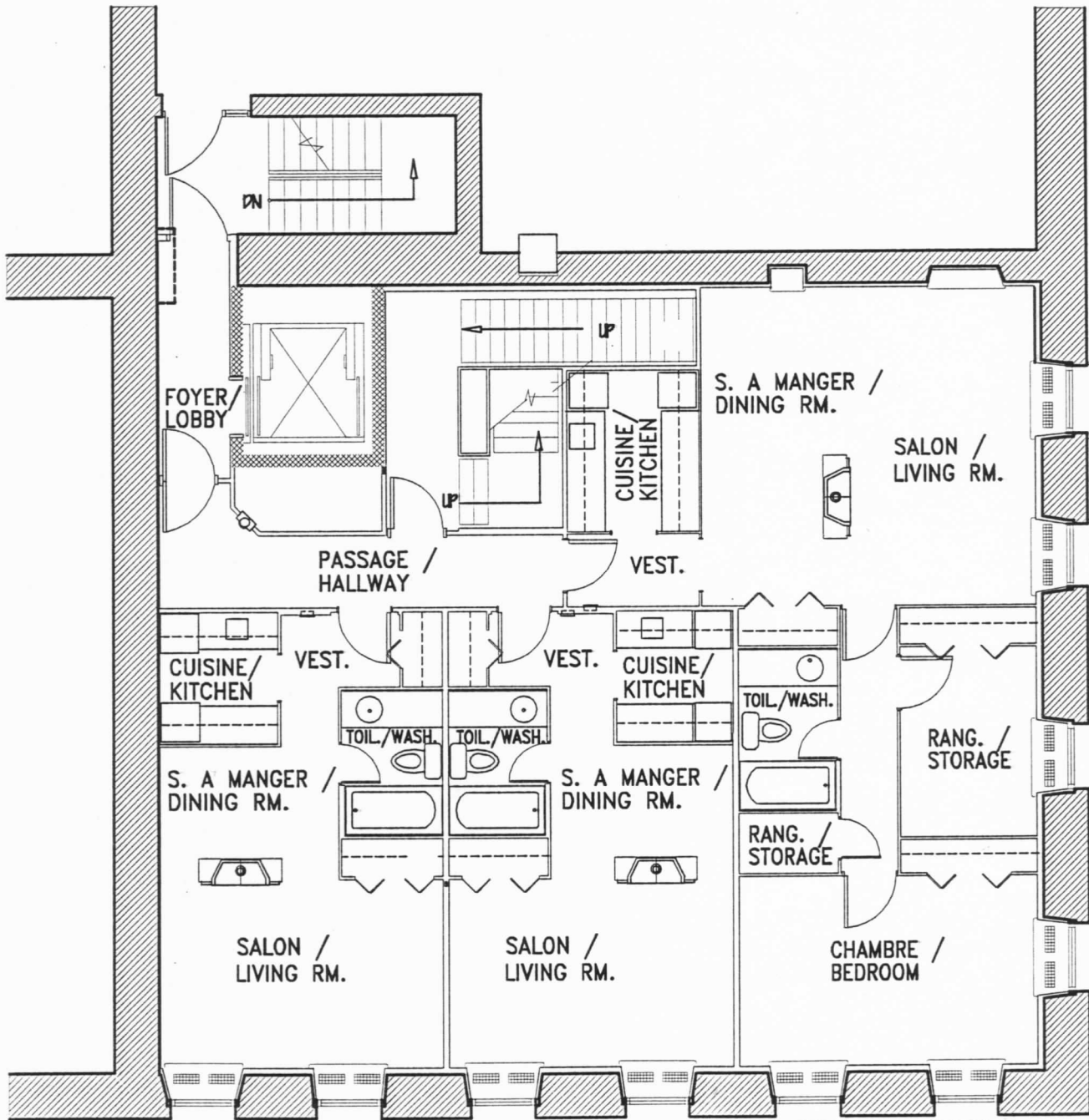
PLAN DU DEUXIÈME ÉTAGE / SECOND FLOOR PLAN
